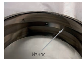
Износ. Поверхность дорожки качения внешнего кольца
