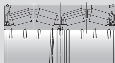
Четырехрядные конические роликоподшипники Sealed-Clean™ увеличенной грузоподъемности – Серия KVS
