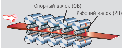
Стан холодной прокатки типа «тандем»
